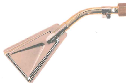
4550 BOQUILLA CON LLAMA PLANA (210 g/h) / FLAT FLAME BURNER (210 g/h) - Para el decapado de pinturas sobre madera y metal, para quemar rastrojos, encendido de barbacoas, deshielo de canalizaciones, instalación de baldosas de plástico... / Suitable for paint scaling on wood and metal, weeding out, and setting fire to barbecues, piping defrosting, plastic tiles installation...
