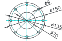
MES30-50 MDS30-50
