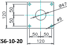
MES6-10-20 MDS6-10-20
