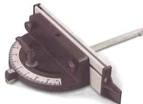
Limitador de ángulo HBS 351-2
